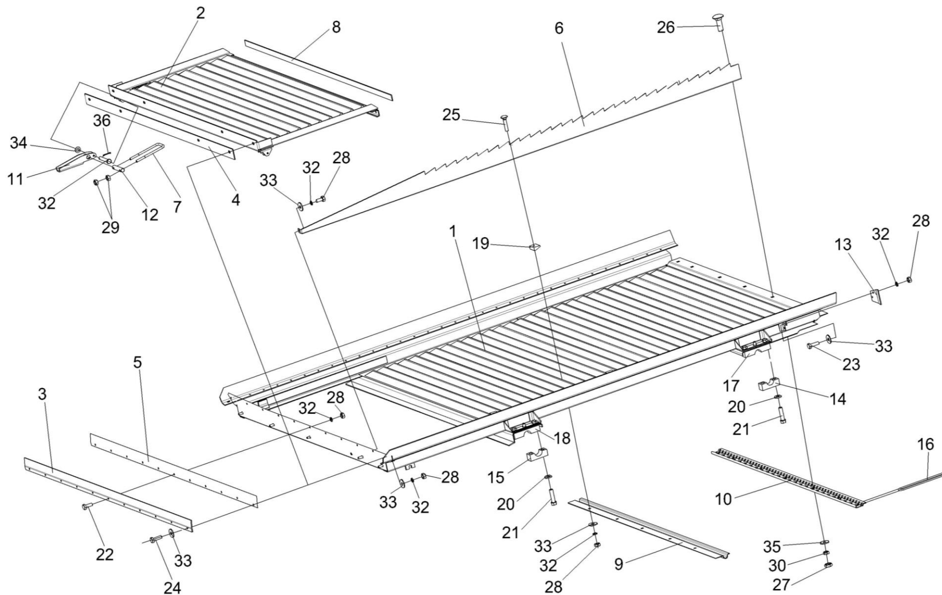
Рисунок 43 – Доска стрясная КЗК-12-0280200
