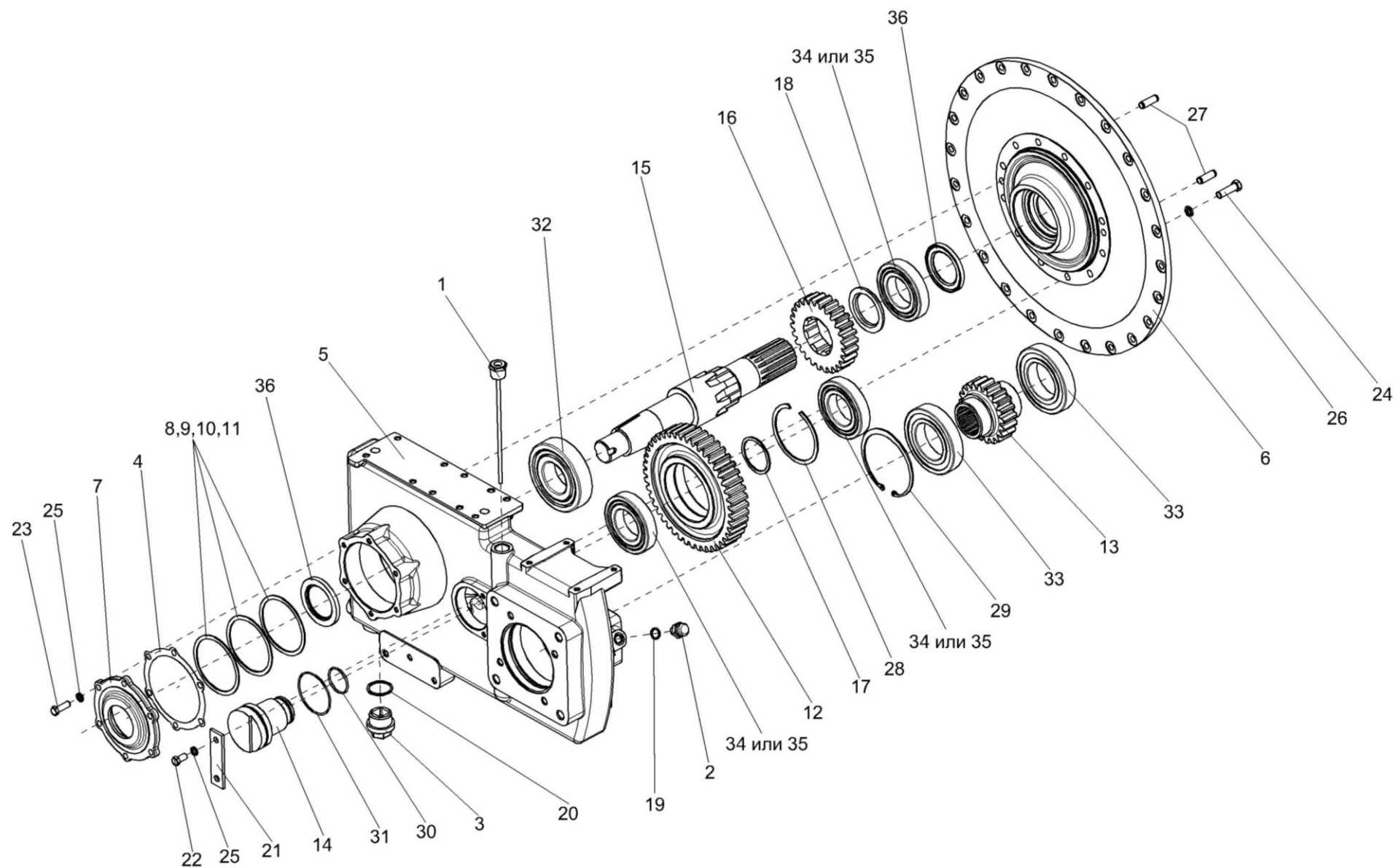
Рисунок 210 – Мультипликатор КЗК-12-0114000
