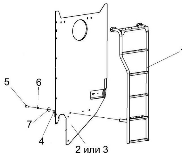
Рисунок 193 – Панель КЗК-12-0128660А
