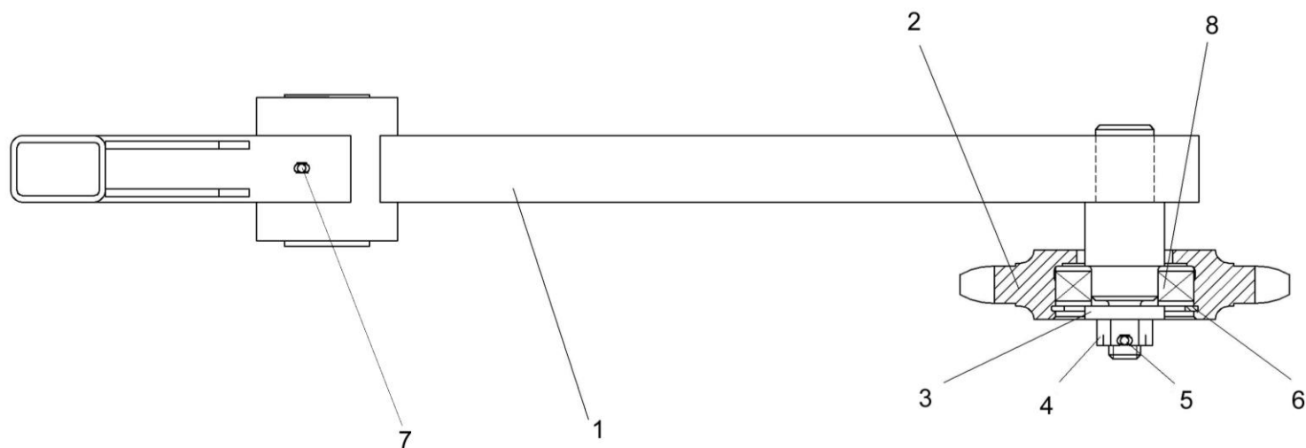
Рисунок 246 – Рычаг КЗК-10-0100680А
