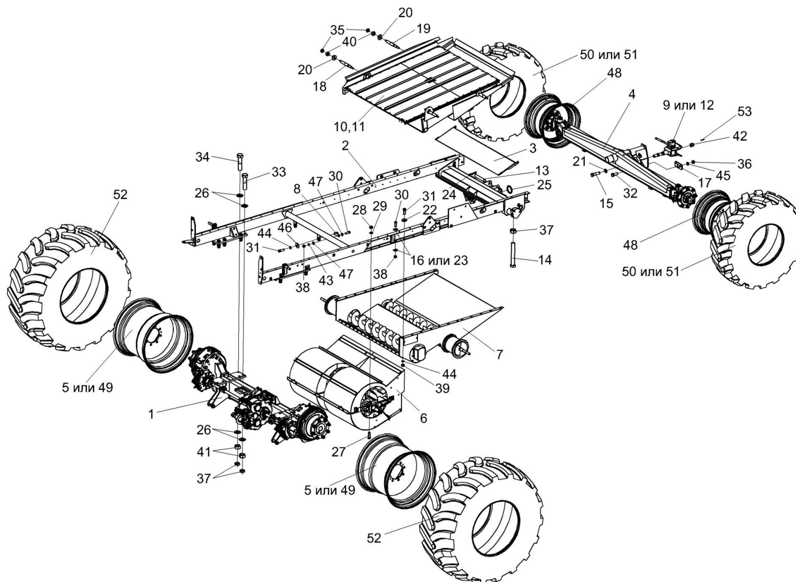
Рисунок 75 – Шасси КЗК-12-0111000В
