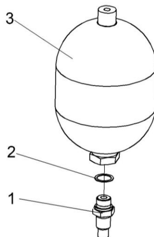
Рисунок 273 – Пневмогидроаккумулятор УЭС-7-0602470
