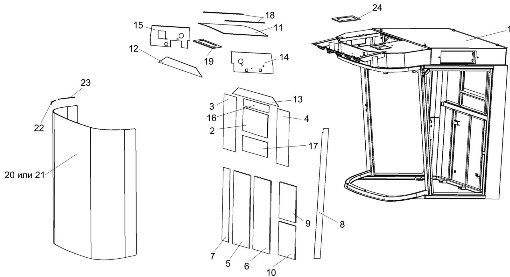
Рисунок 145 – Каркас КЗК-12-0120010
