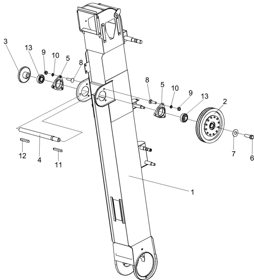
Рисунок 118 – Элеватор зерновой КЗК-10-0214000-01 (лист 1)
