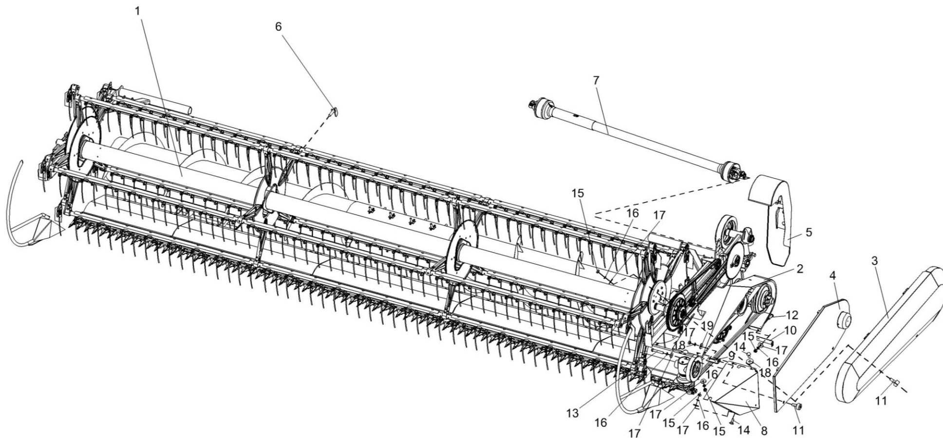
Рисунок 1 – Жатка для зерновых культур ЖЗК-7-2 КЗР 1500000-23
