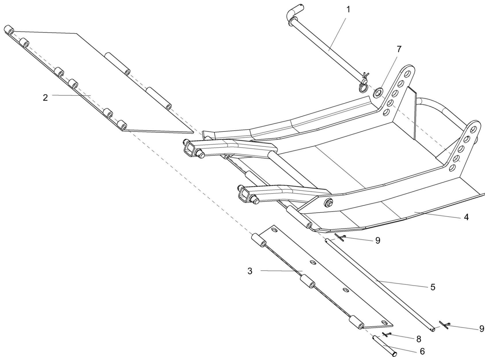
Рисунок 5 – Башмак K3P 1516200
