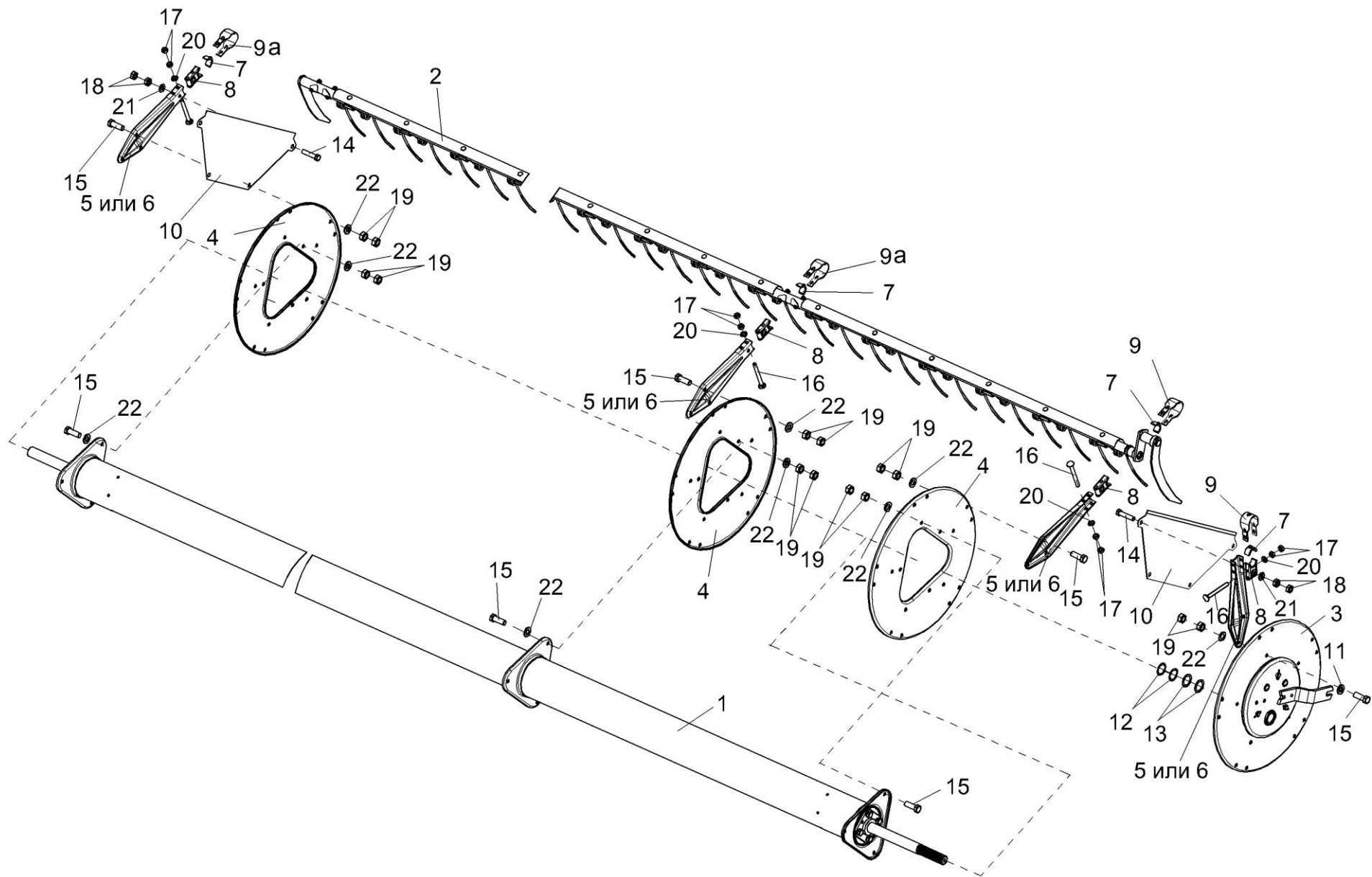
Рисунок 26 – Мотовило КЗР 1573500
