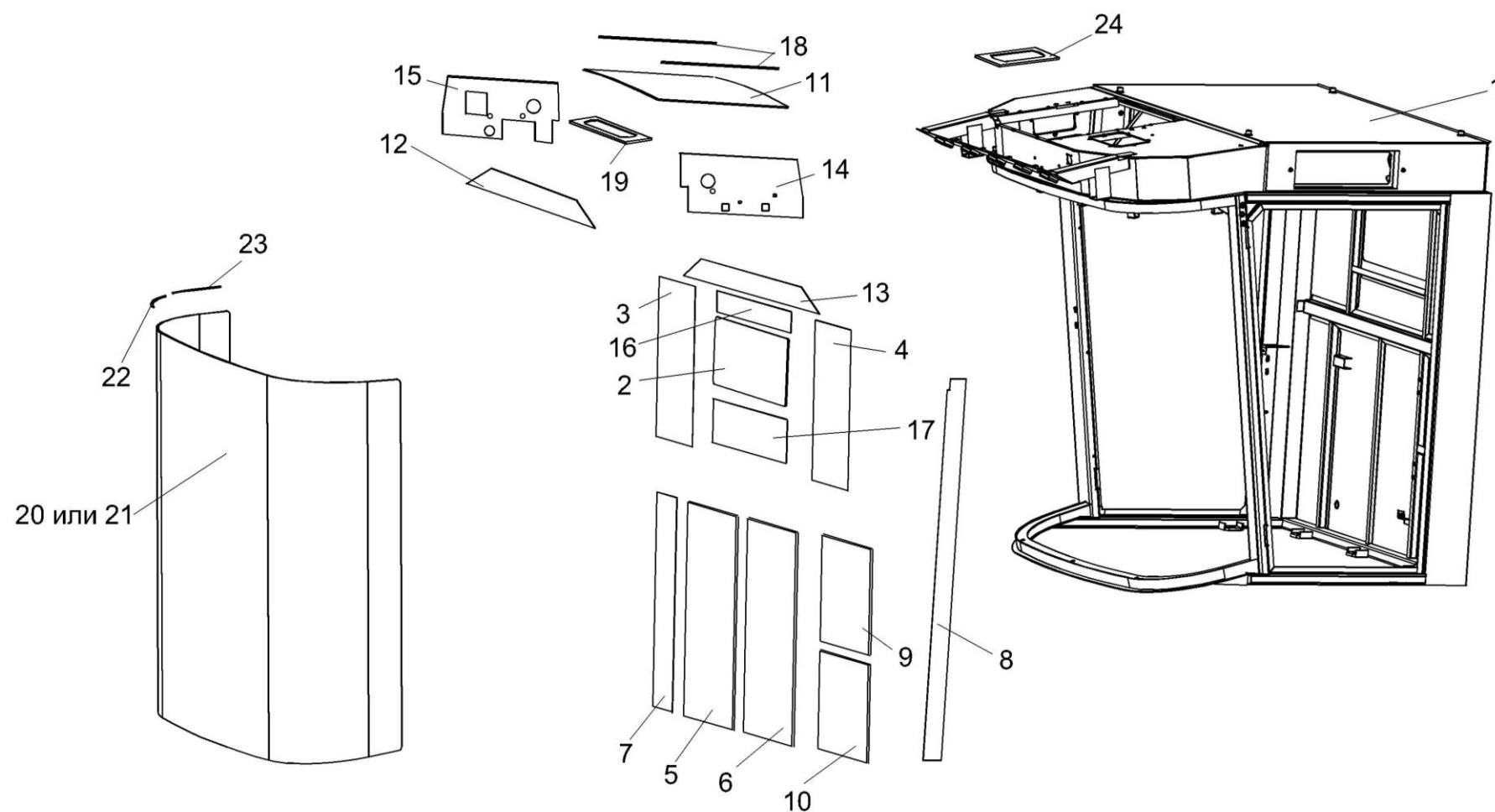
Рисунок 149 – Каркас КЗК-12-0120010
