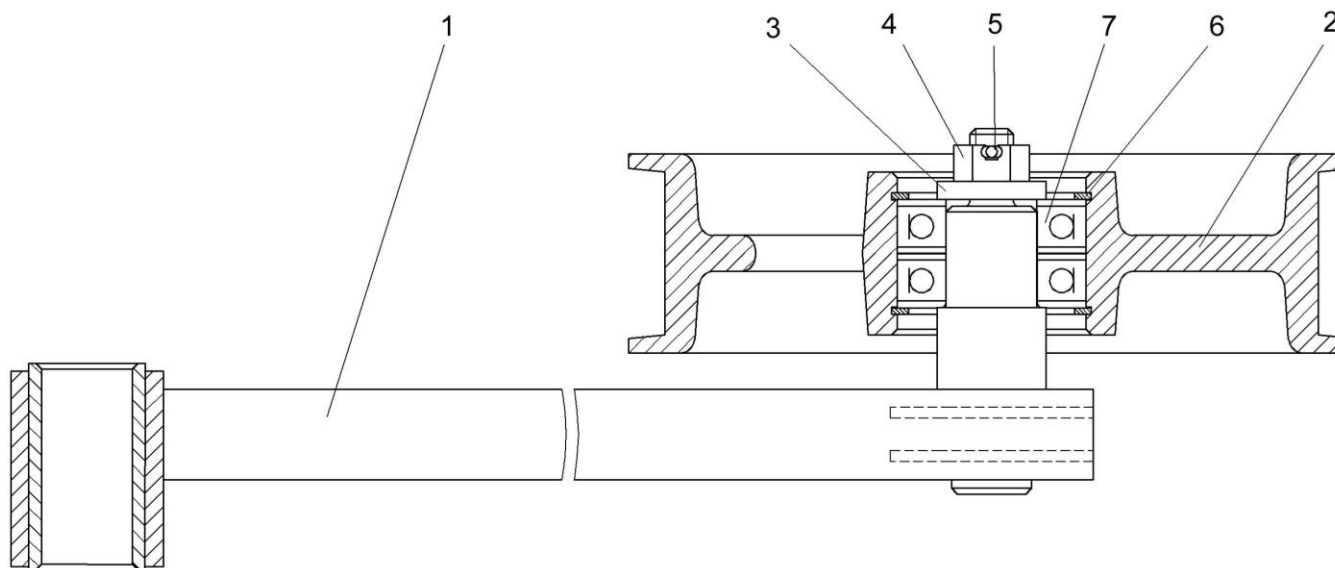
Рисунок 252 – Рычаг КЗК-10-0100620
