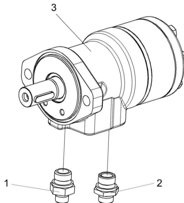
Рисунок 20 – Гидромотор КЗК-12-1790990А
