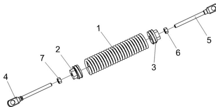
Рисунок 246 – Пружина КЗК-12-3-0220050
