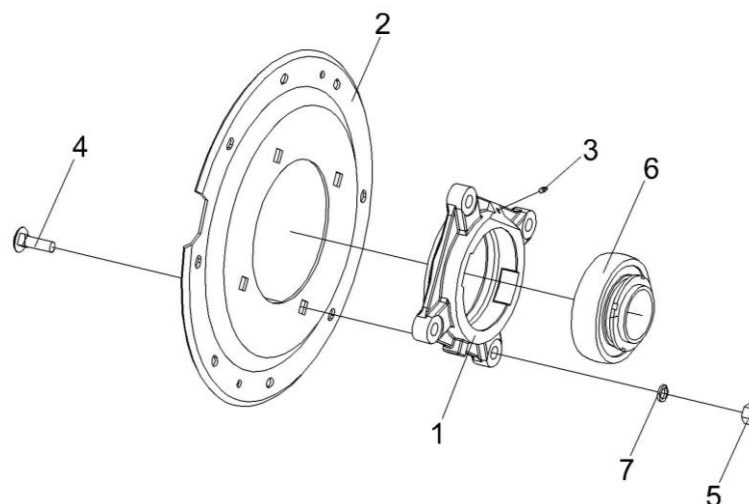
Рисунок 67 – Фланец КЗК-10-0102070
