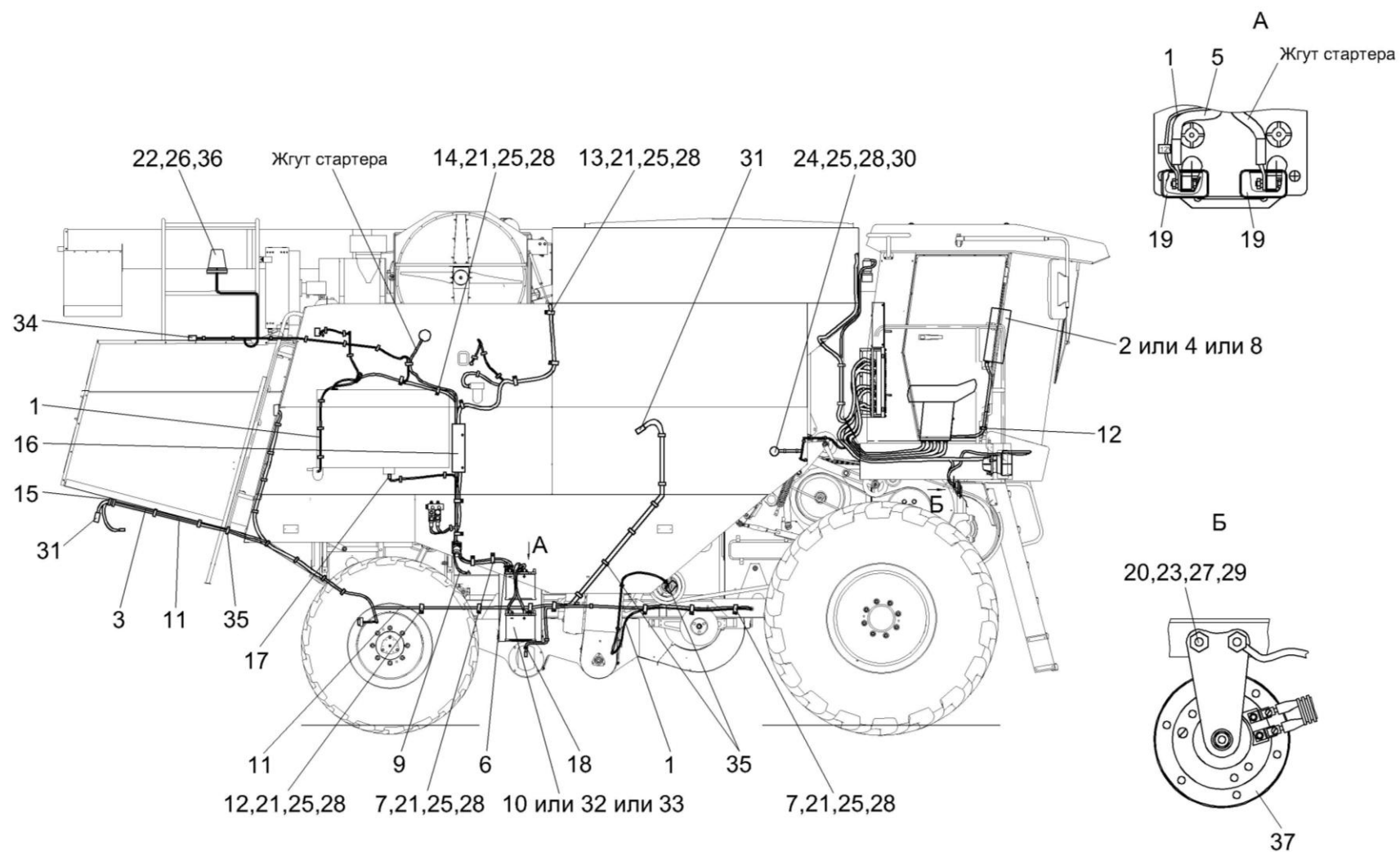
Рисунок 7 – Электрооборудование молотилки самоходной КЗК-12-0100000Б-12 (лист 2)
