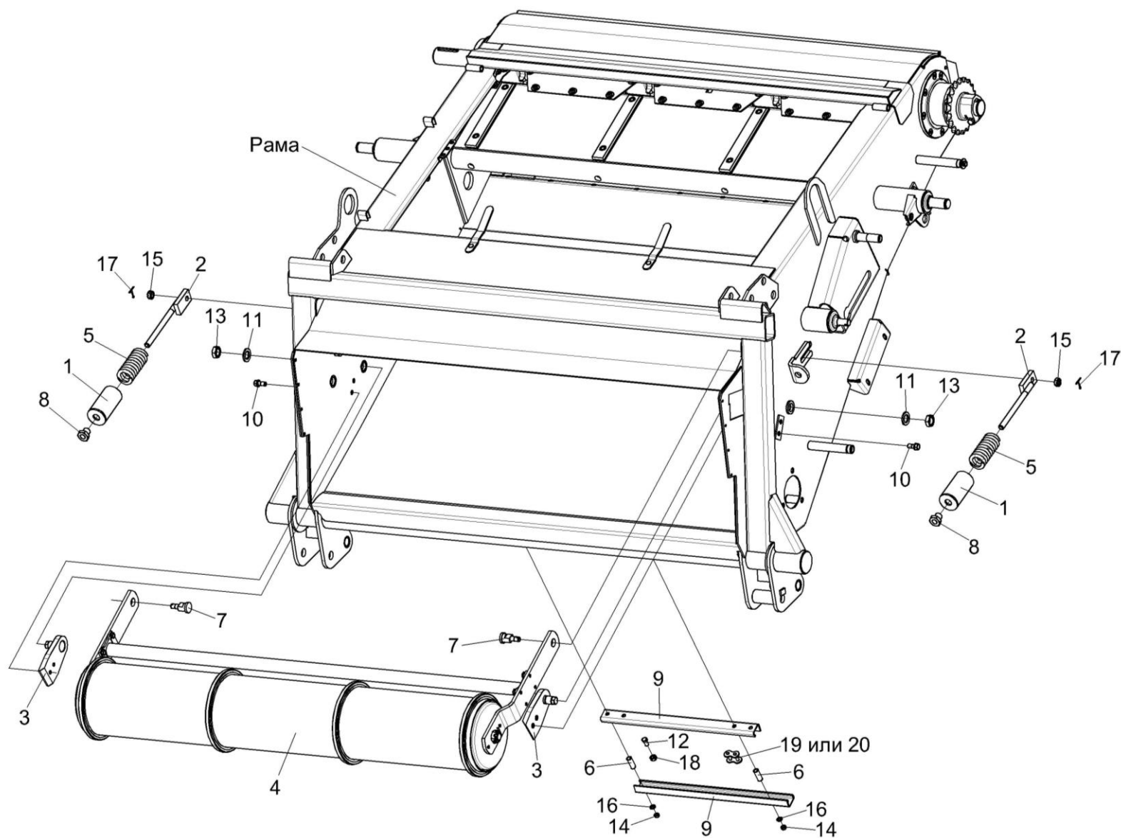
Рисунок 22 – Установка вала нижнего КЗК-12-1816000В
