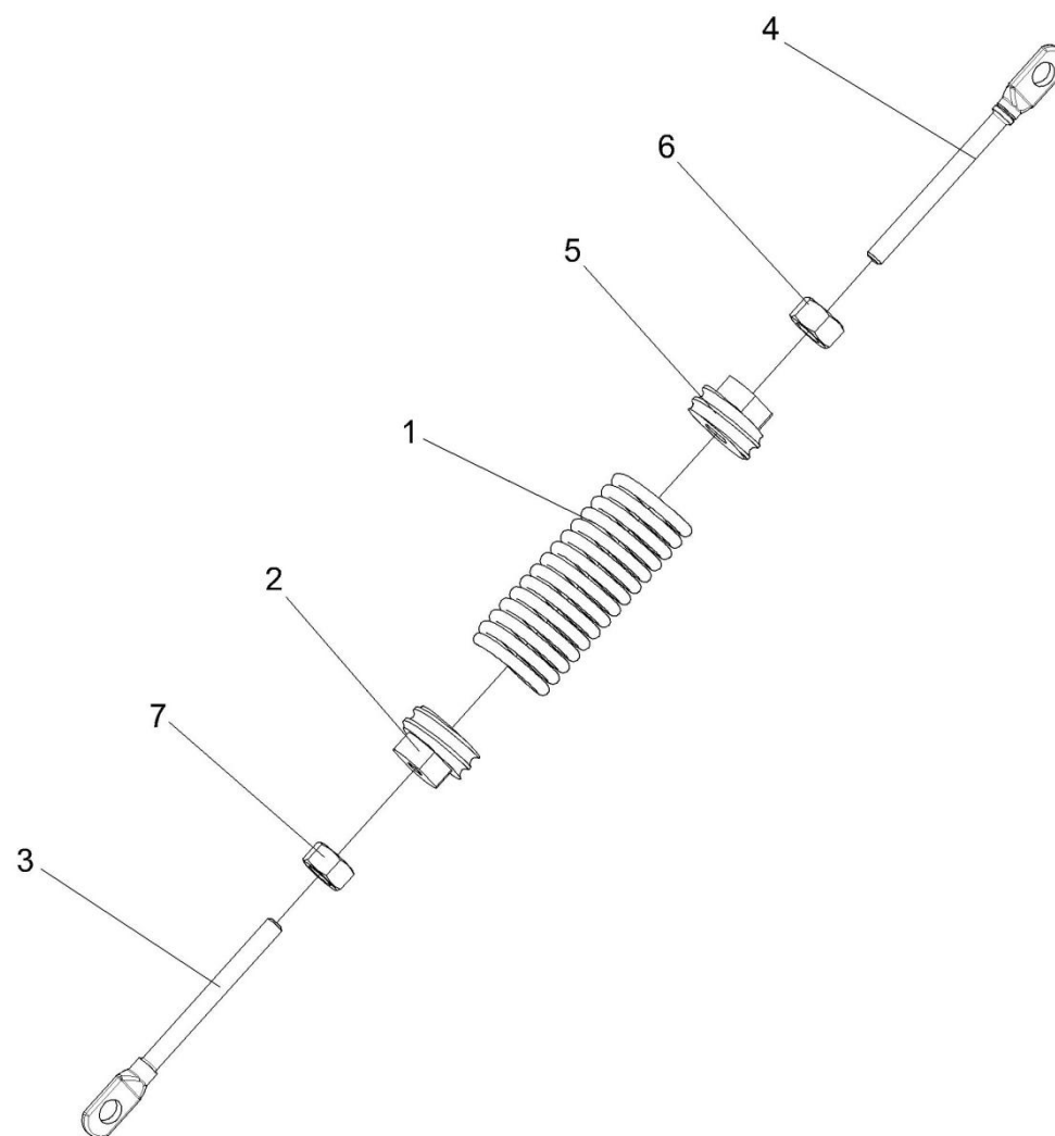
Рисунок 132 – Пружина КЗК-12-0221140А
