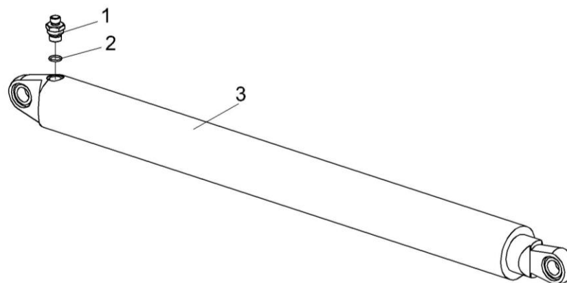
Рисунок 273 – Гидроцилиндр КЗК-12-0602740
