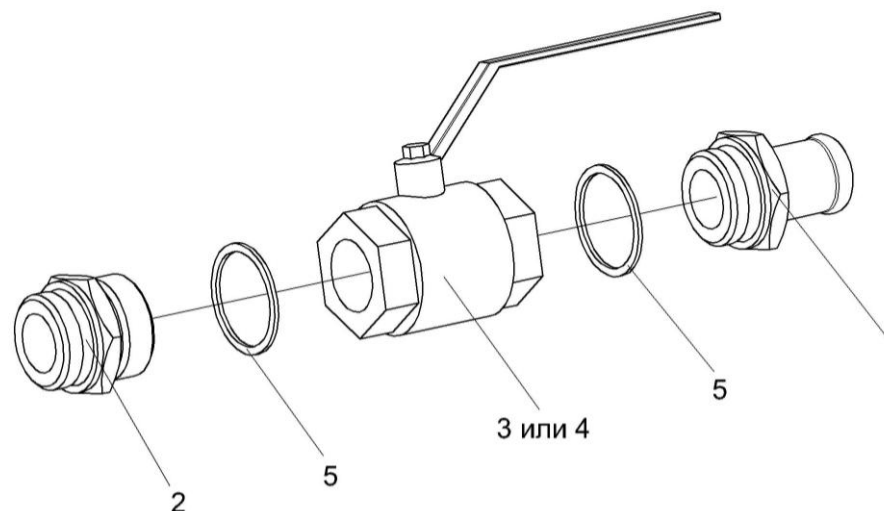
Рисунок 277 – Кран КЗК-10-0602380
