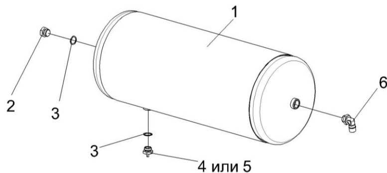
Рисунок 239 – Ресивер КЗК-2-12-0800030
