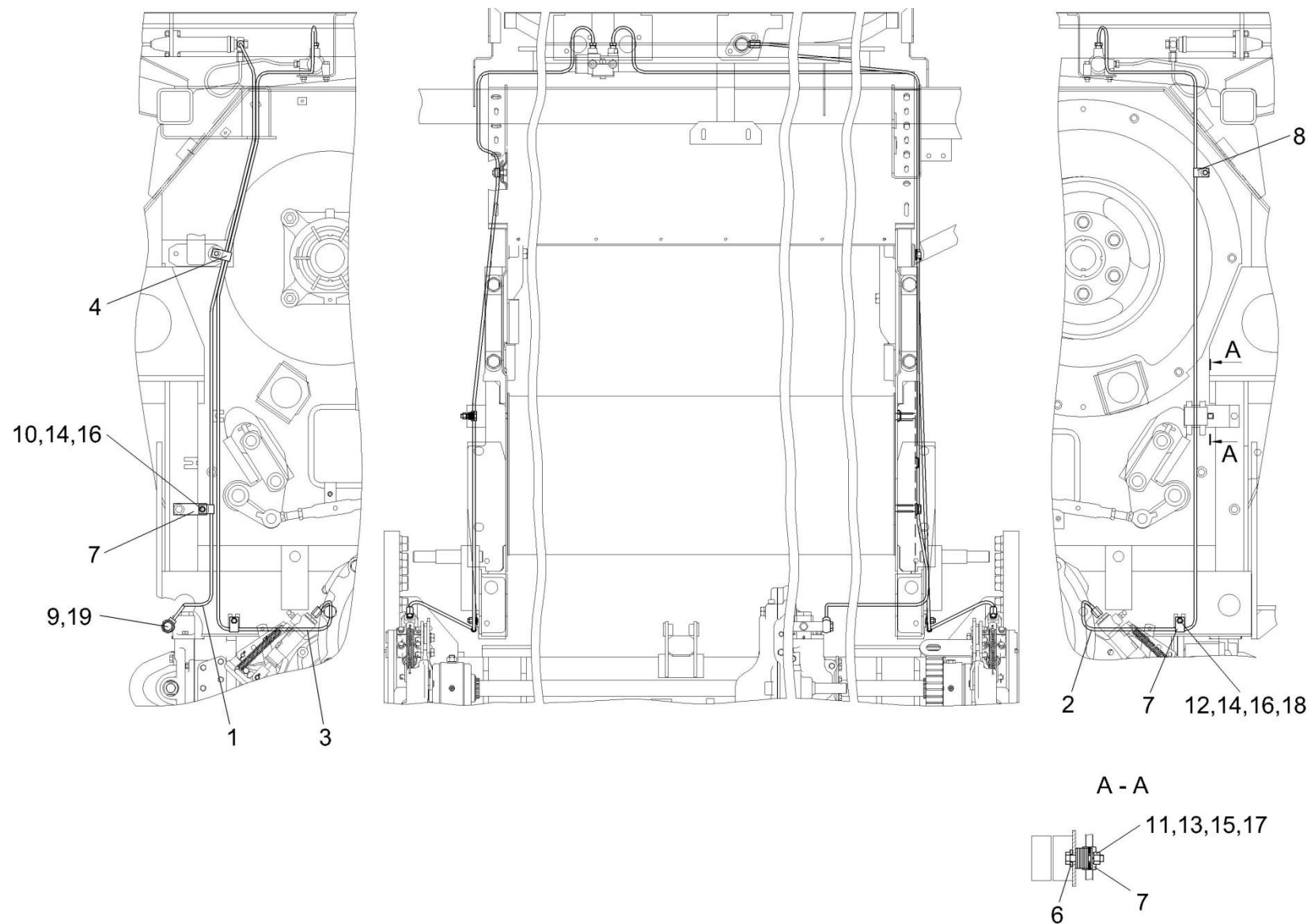
Рисунок 189 – Установка трубопроводов моста ведущих колес КЗК-12-0119630
