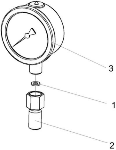
Рисунок 275 – Манометр КЗК-12-0602810
