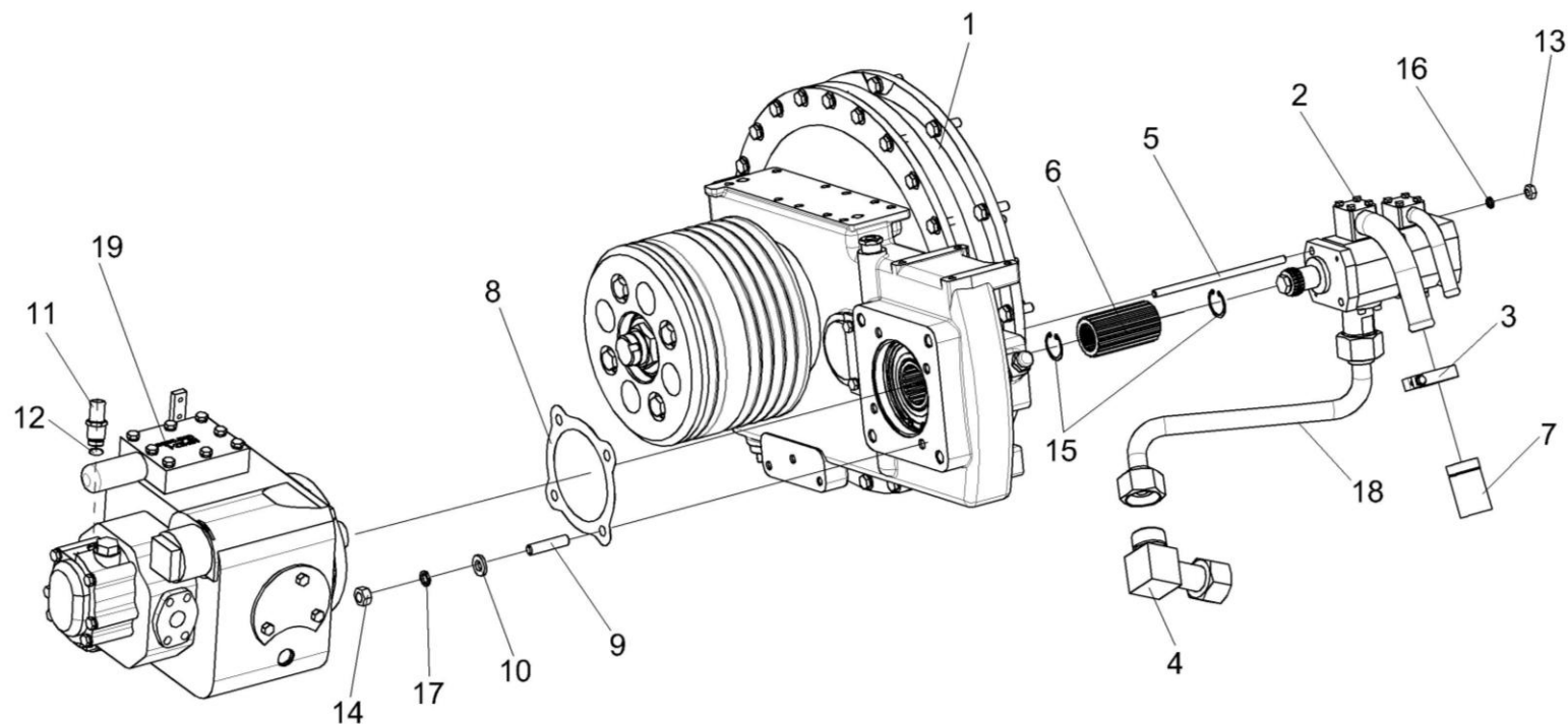
Рисунок 211 – Установка гидронасосов КЗК-12-3-0106740
