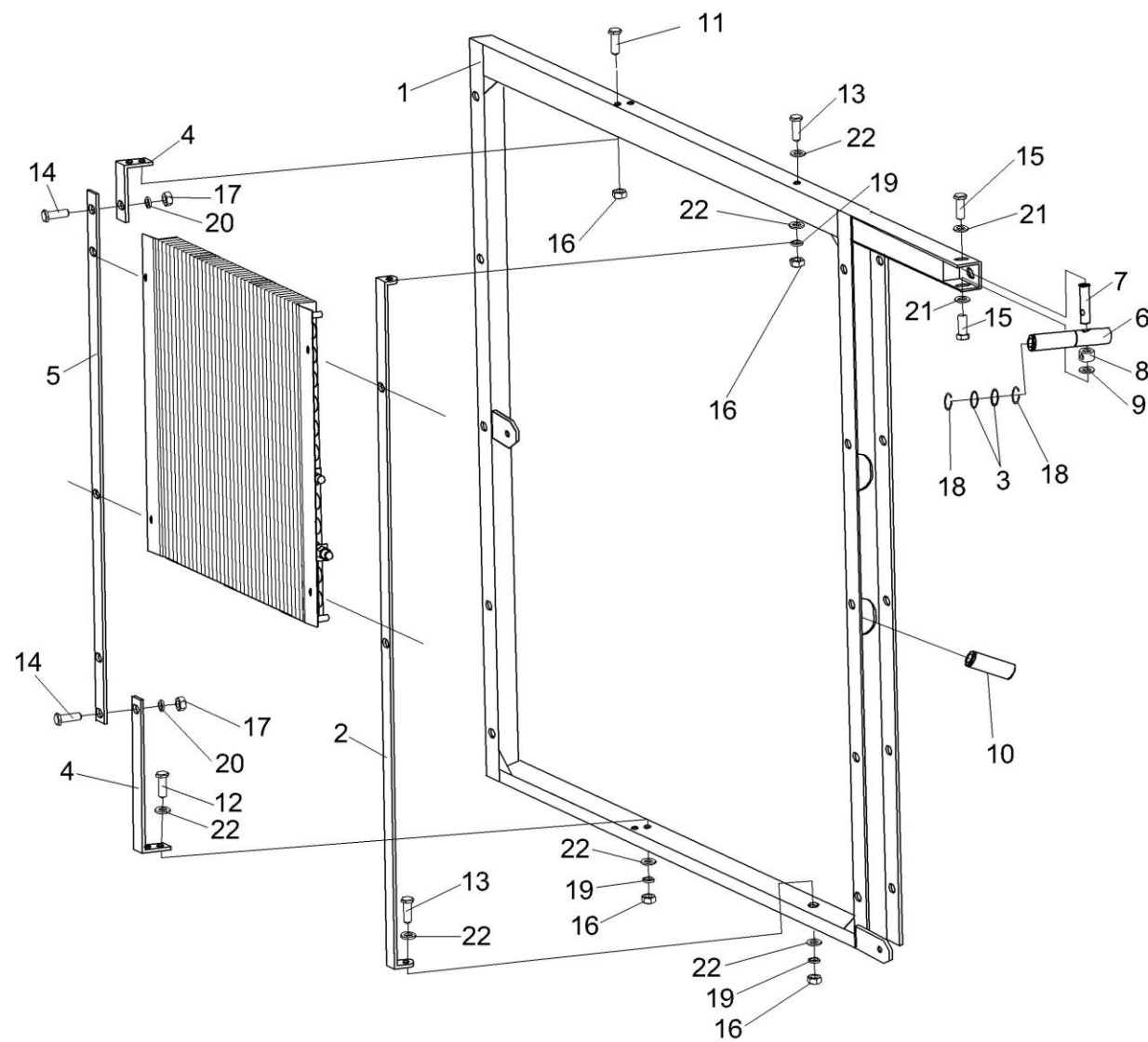
Рисунок 225 – Рама КЗК-12-3-0112080
