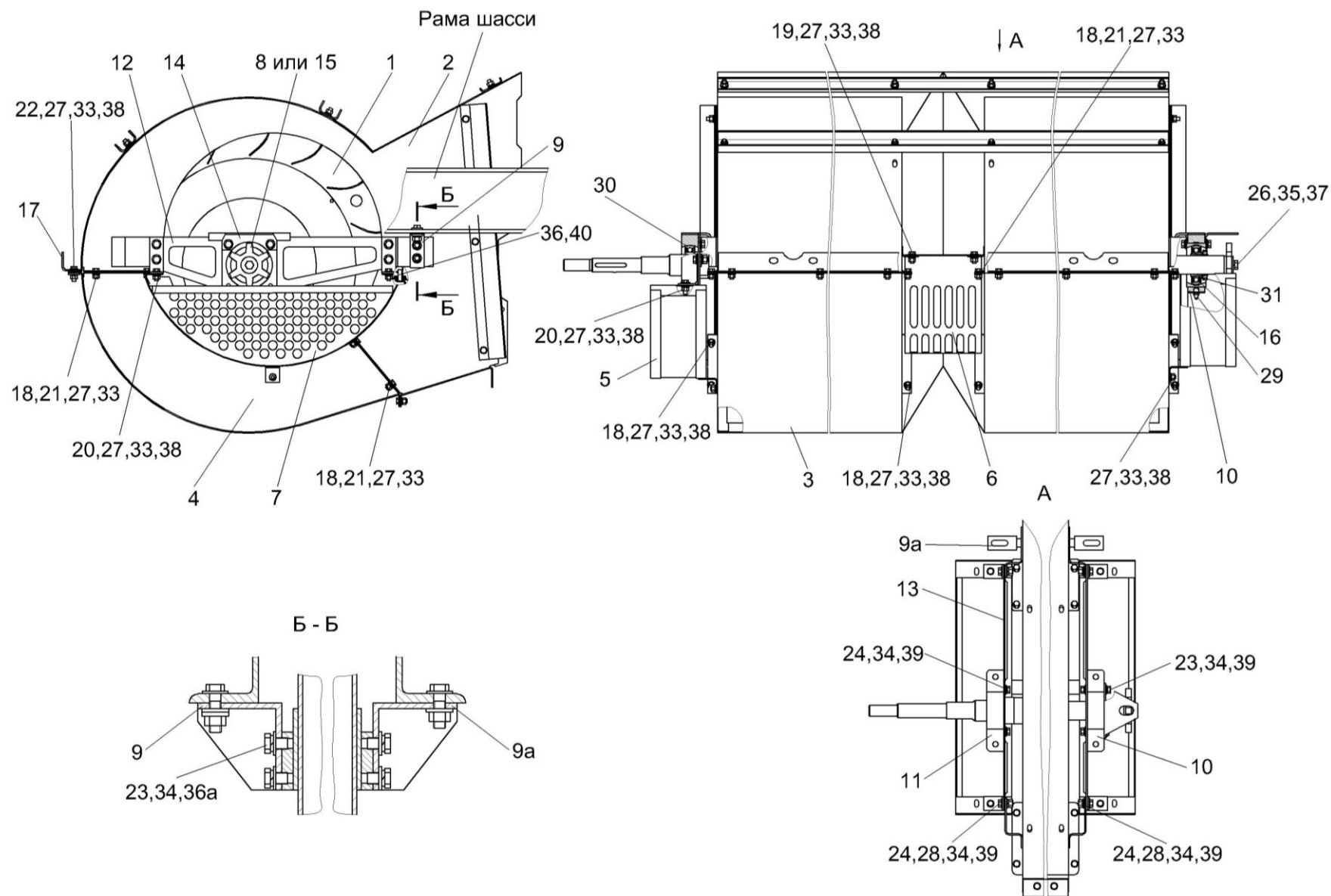
Рисунок 99 – Вентилятор КЗК-10-0217000
