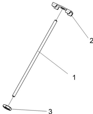
Рисунок 182 – Зажим УЭС 0302540
