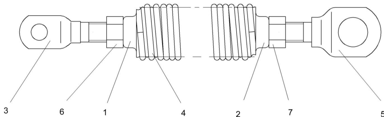
Рисунок 254 – Пружина КЗК-10-0100720А
