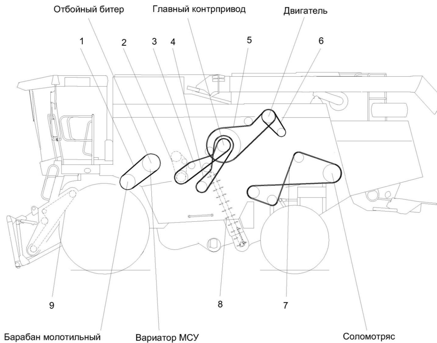
Рисунок 283 – Схема приводов (вид слева)
