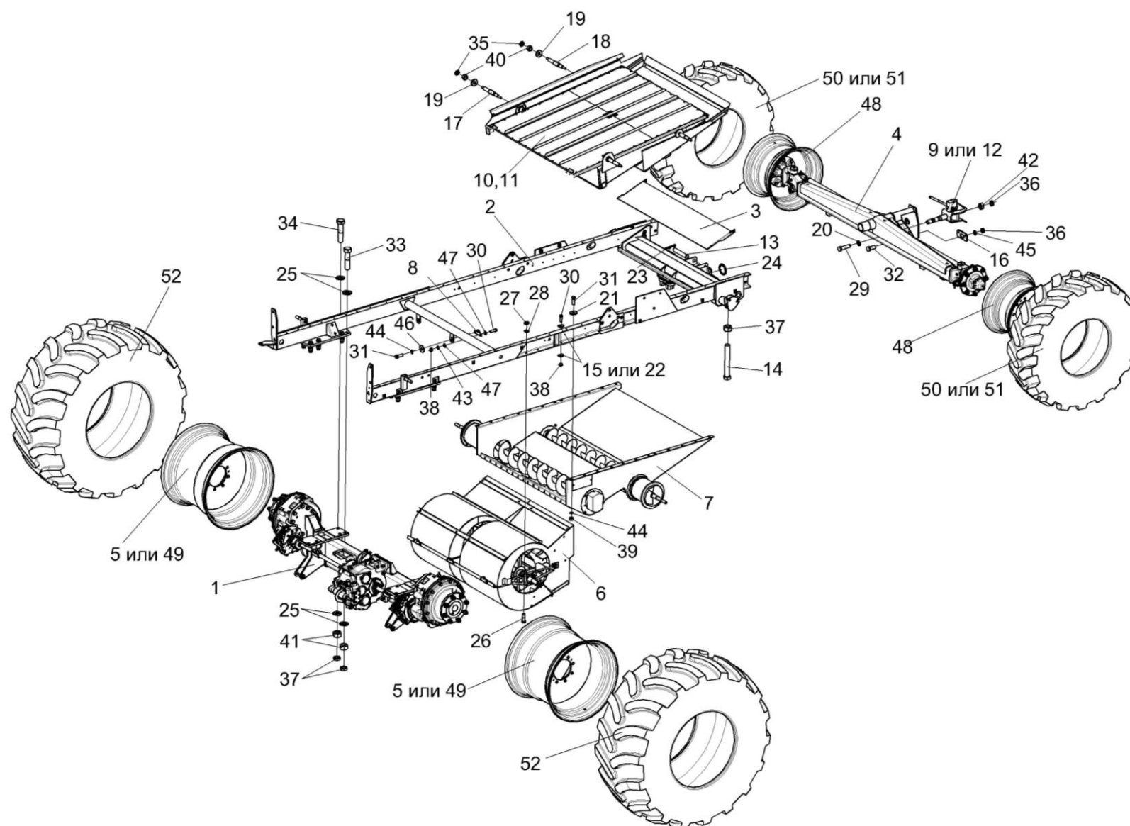
Рисунок 79 – Шасси КЗК-12-0111000В
