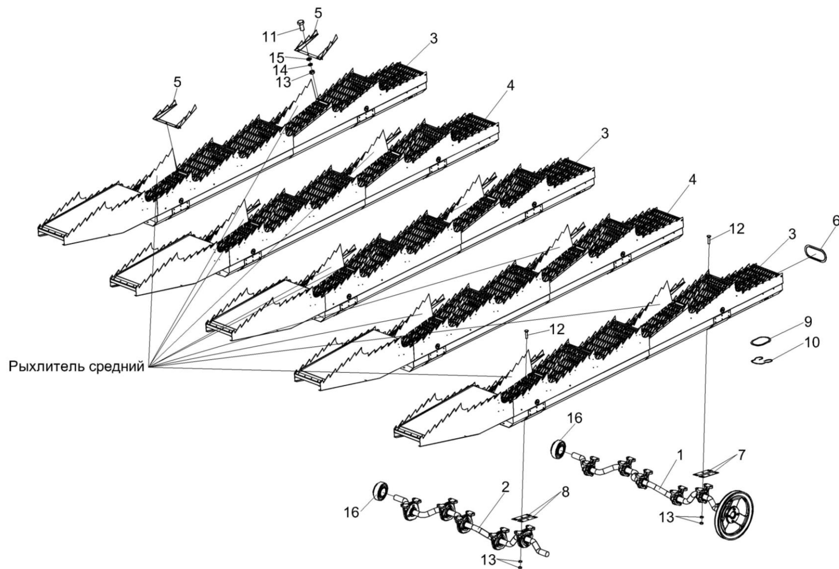
Рисунок 68 – Соломотряс КЗК-12-0212040
