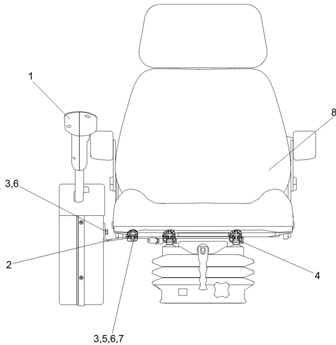
Рисунок 166 – Сиденье КЗК-12-0119290Б-01
