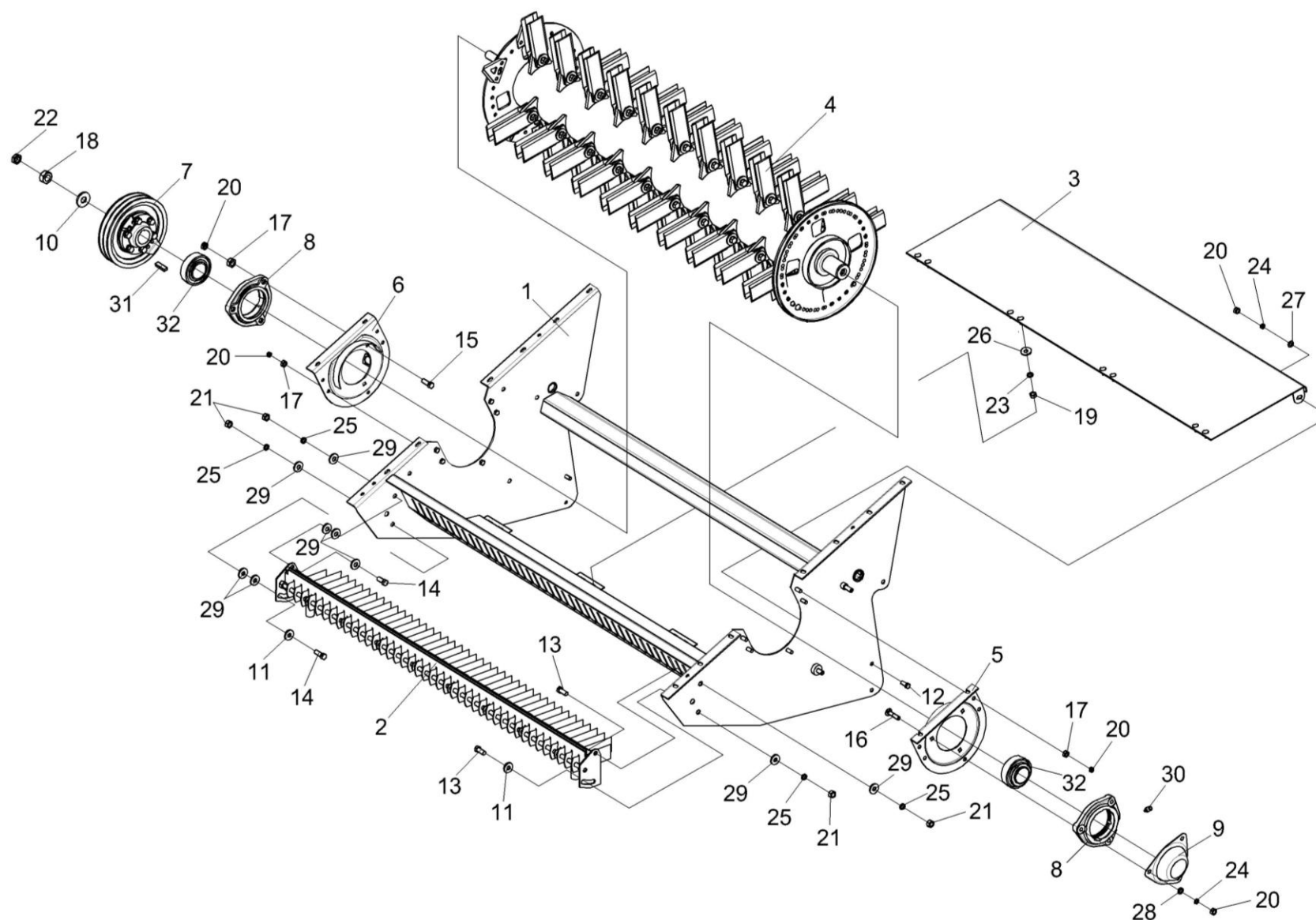
Рисунок 135 – Соломоизмельчитель КЗК-10-0290000А
