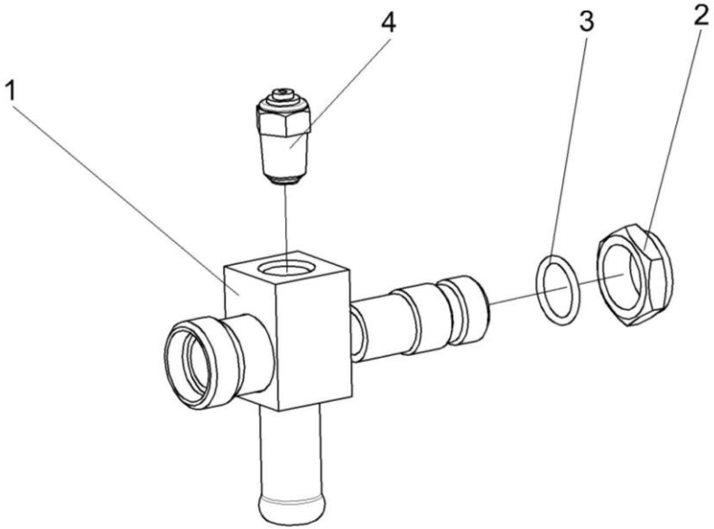
Рисунок 259 – Крестовина КЗК-12-0601330
