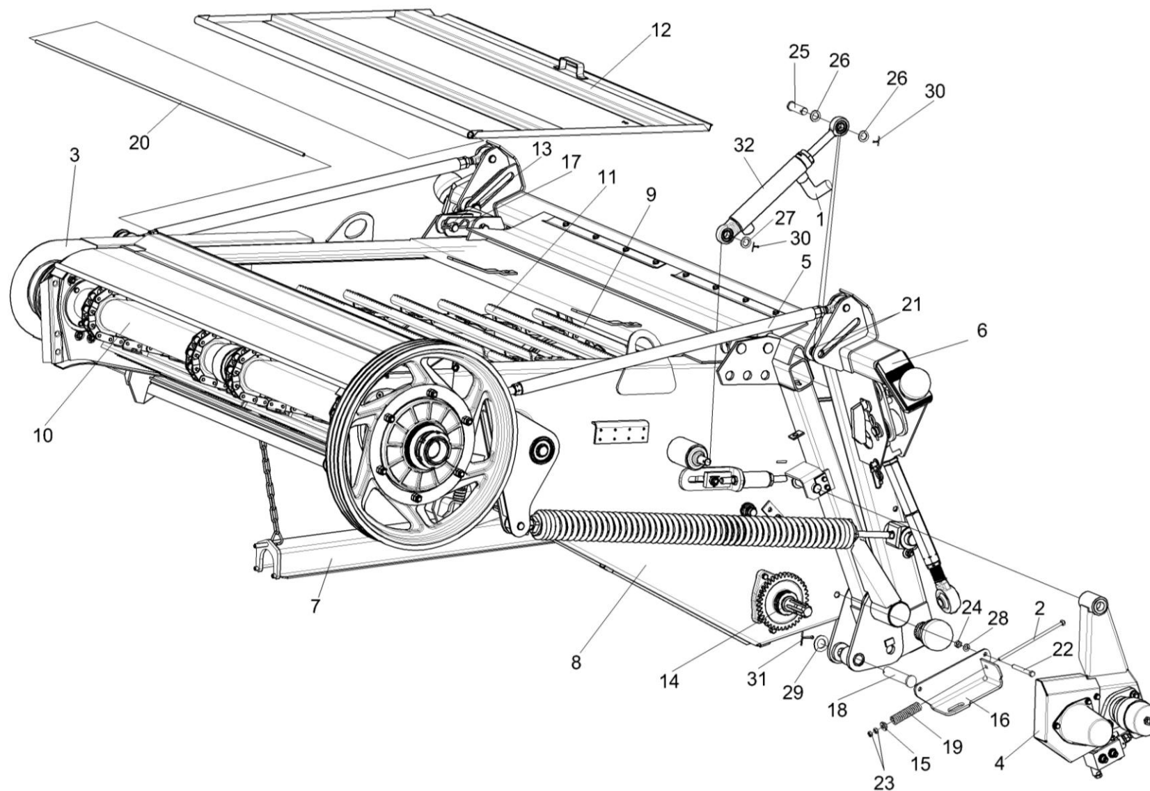
Рисунок 11 – Камера наклонная КЗК-12-1810000В
