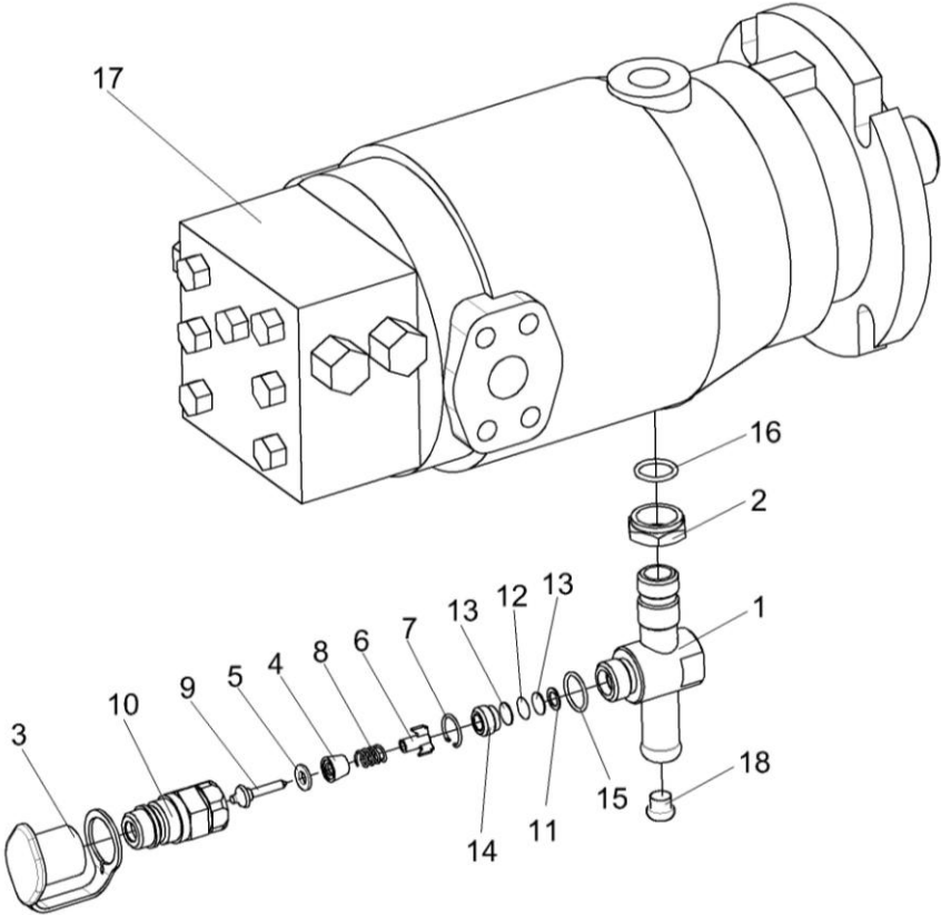
Рисунок 260 – Гидромотор КЗК-12-0601500-01
