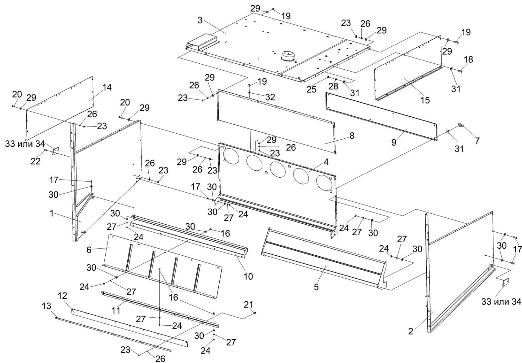
Рисунок 236 – Капот КЗК-2-12-0228300
