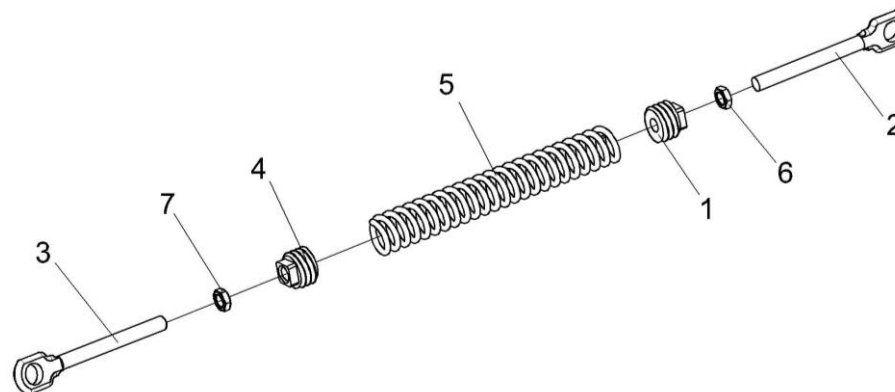
Рисунок 222 – Пружина КЗК-12-3-0126640
