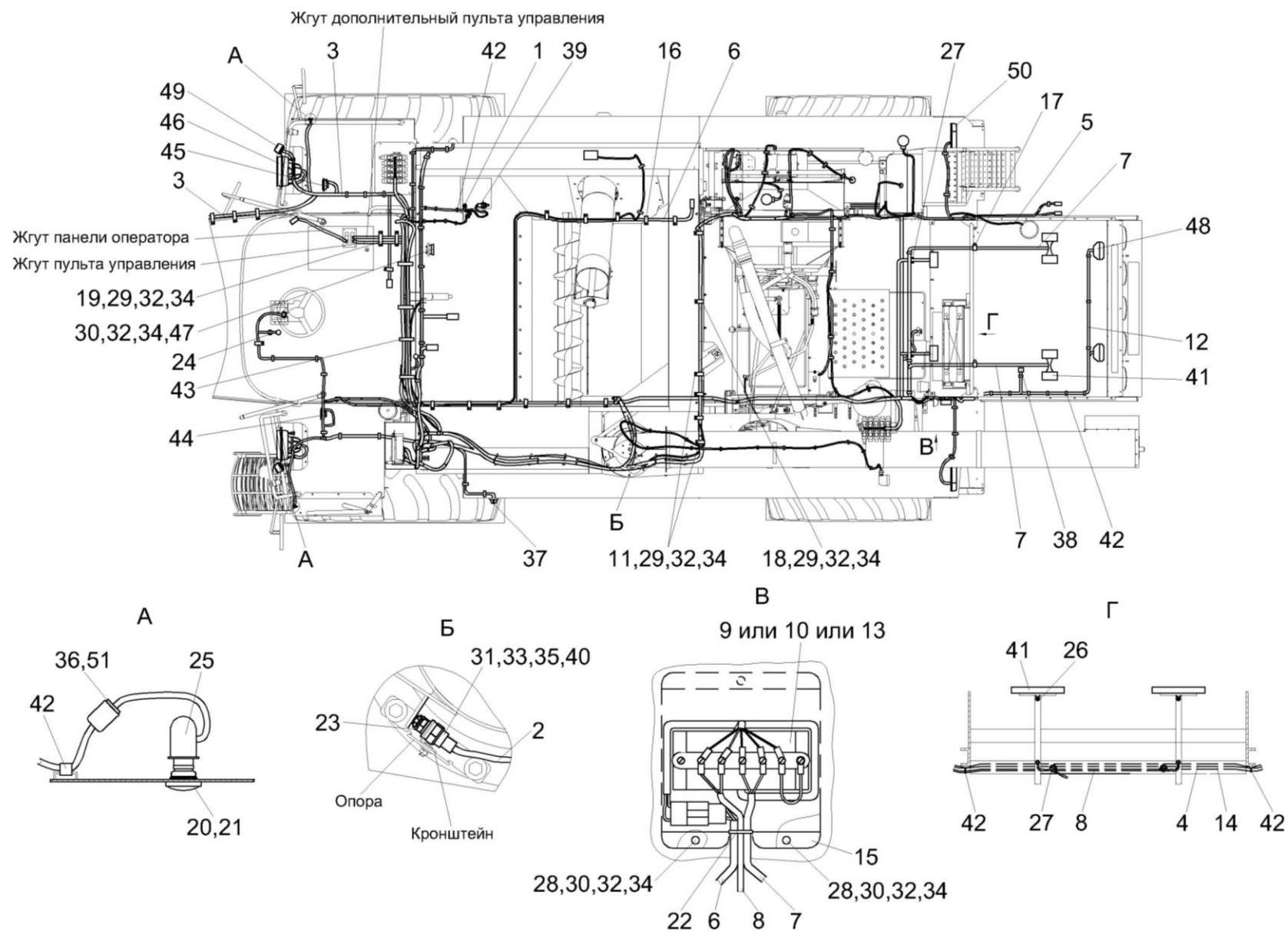
Рисунок 8 – Электрооборудование молотилки самоходной КЗК-12-0100000Б-12 (лист 3)
