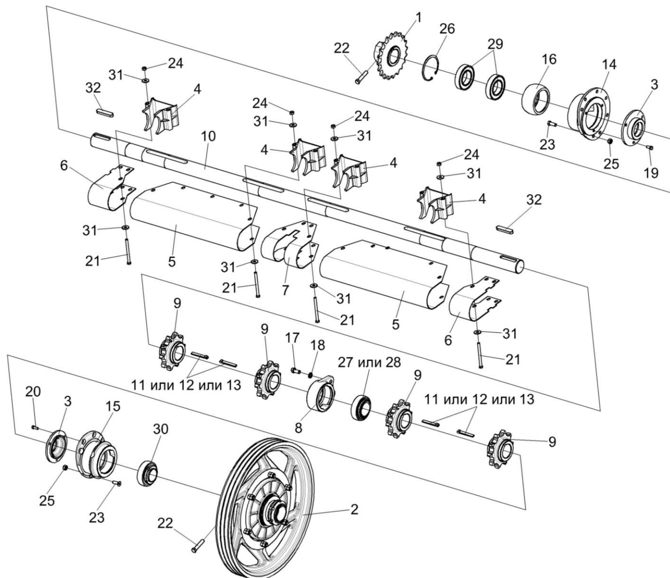
Рисунок 14 – Установка вала верхнего КЗК-12-1813000Б
