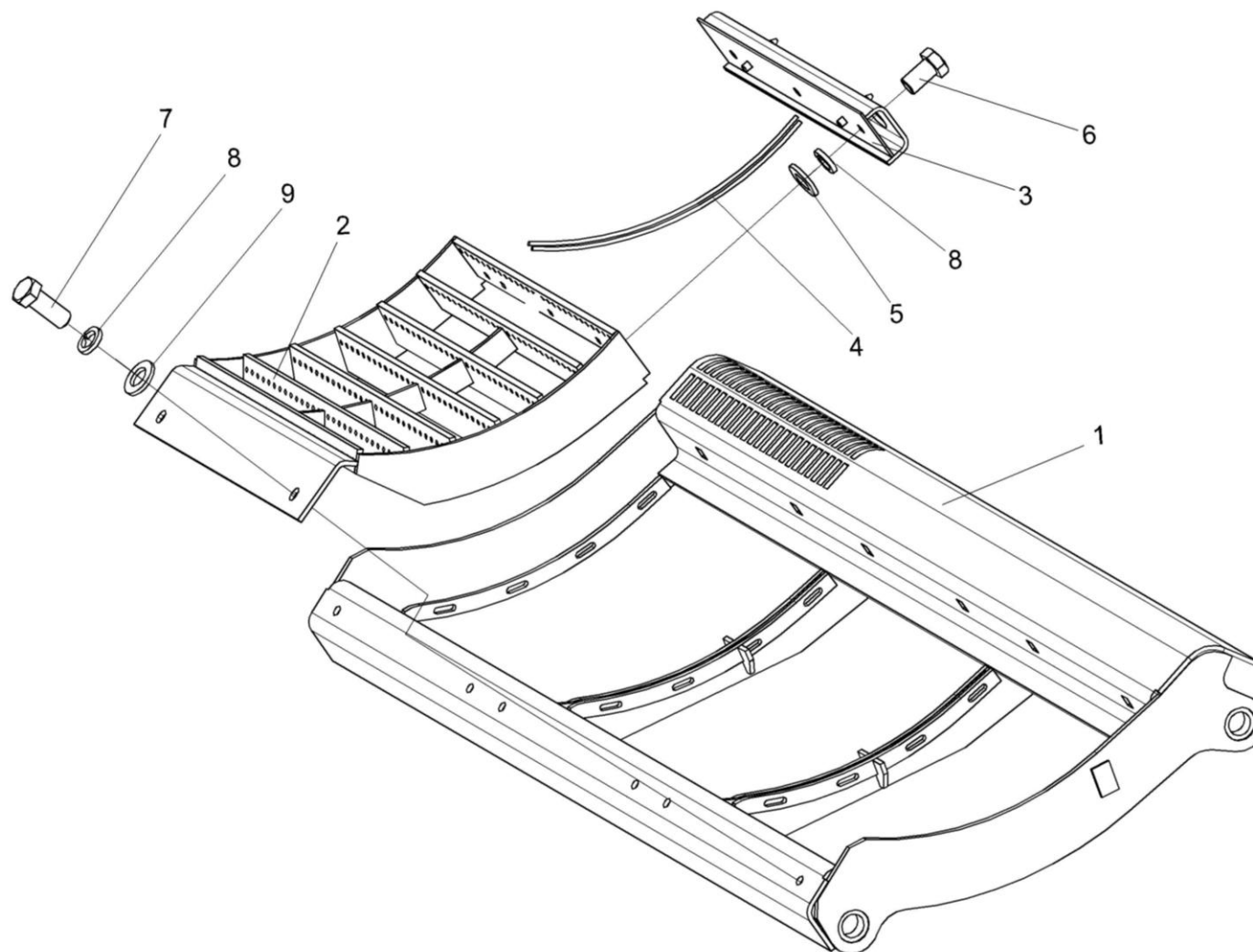
Рисунок 63 – Подбарабанье КЗК-12-0103030
