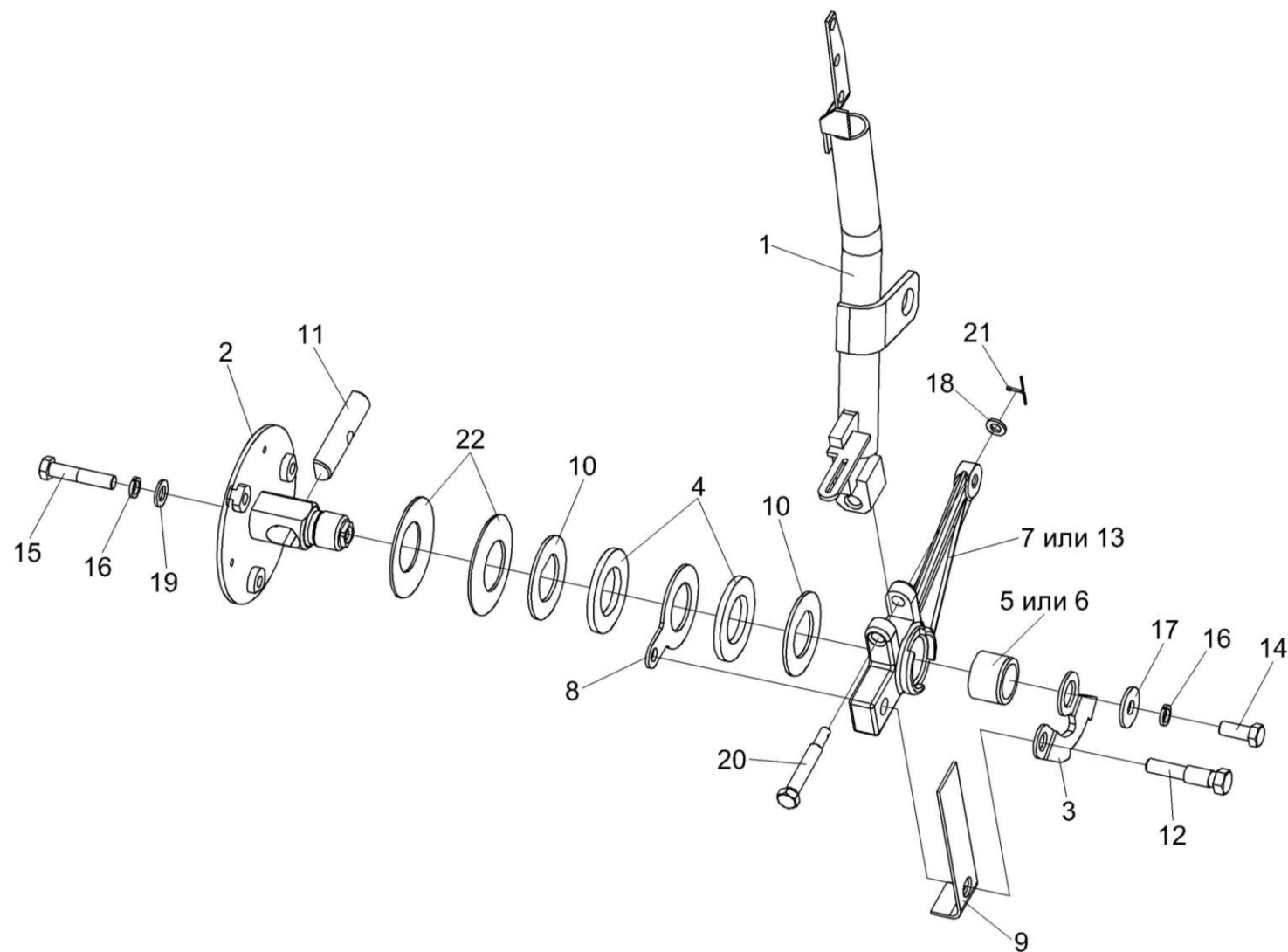
Рисунок 167 – Рычаг КЗК-12-0119920Б
