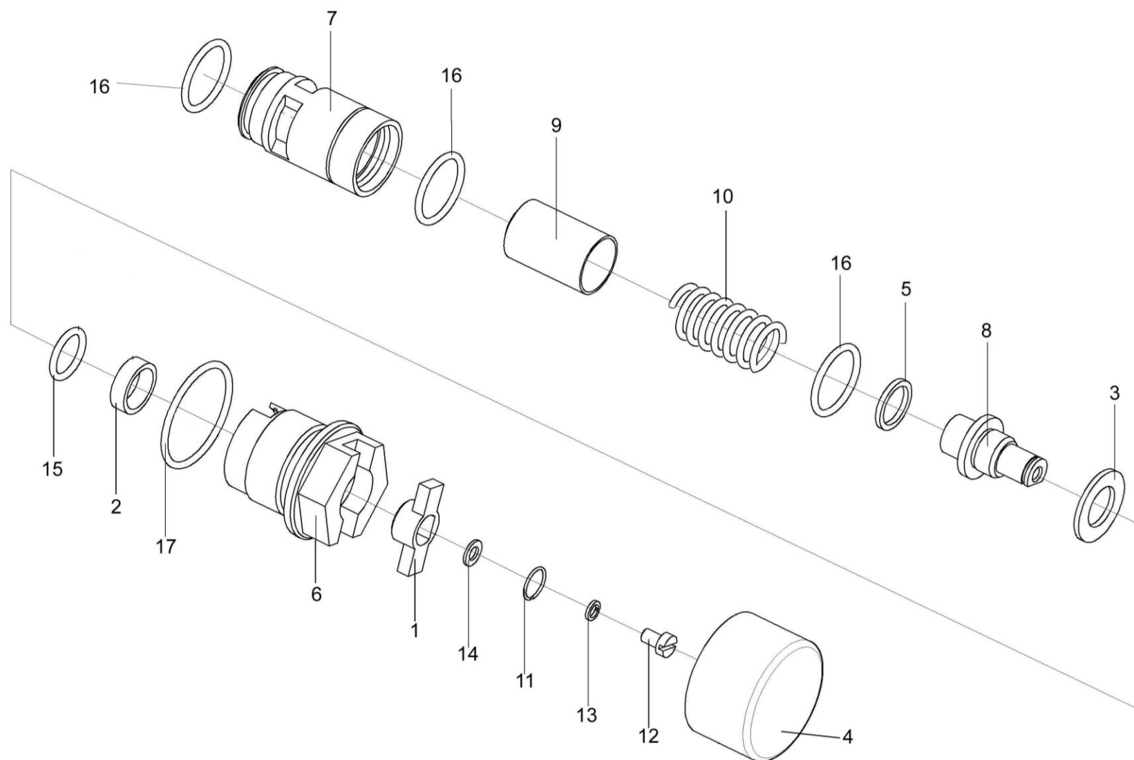
Рисунок 268 – Клапан-сигнализатор УЭС 0603660-01
