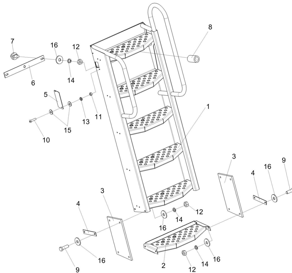
Рисунок 193 – Трап КЗК-12-0117030А
