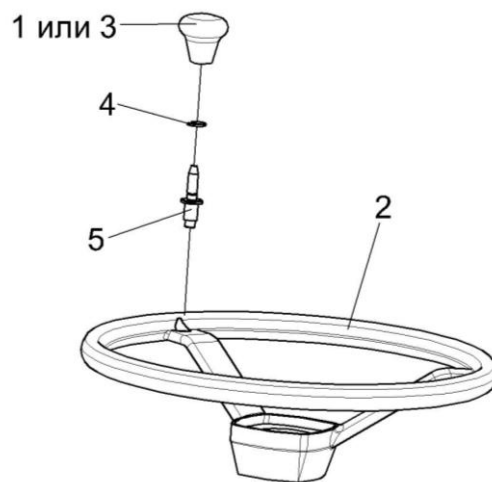
Рисунок 181 – Колесо рулевое УЭС 0302560
