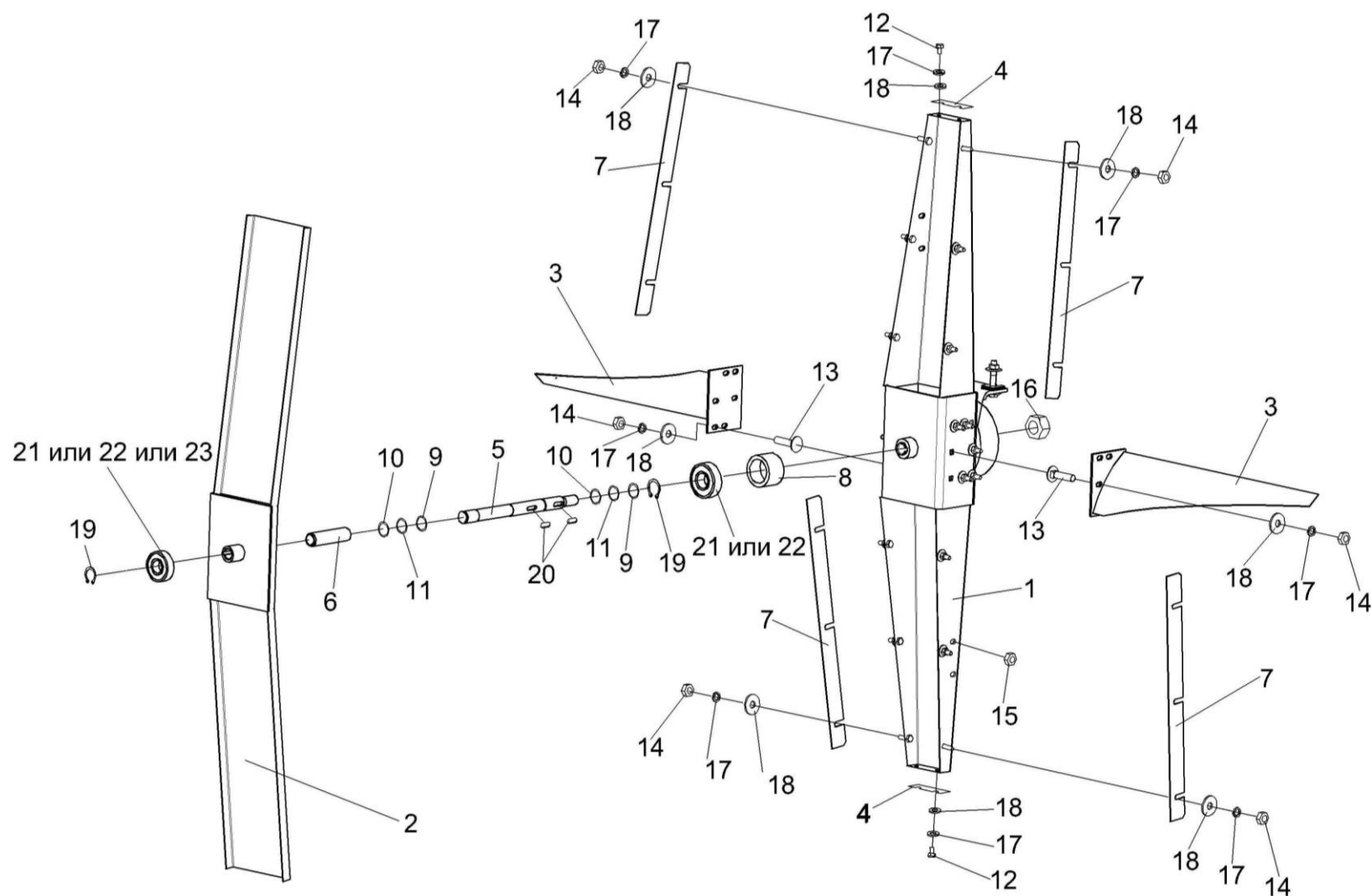
Рисунок 226 – Пылесъемник КЗК-12-3-0112130А
