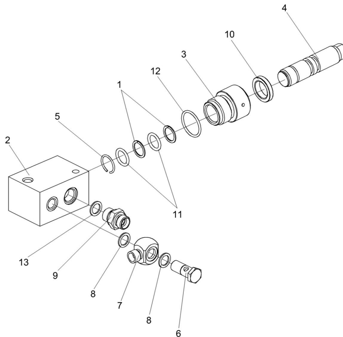
Рисунок 19 – Гидроцилиндр КЗК-12-1790200А
