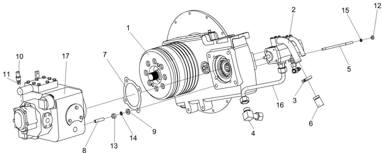
Рисунок 209 – Установка гидронасосов K3K-12-3-0106730
